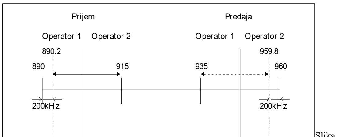
6.12 Raspored frekvencija za dva GSM operatora
