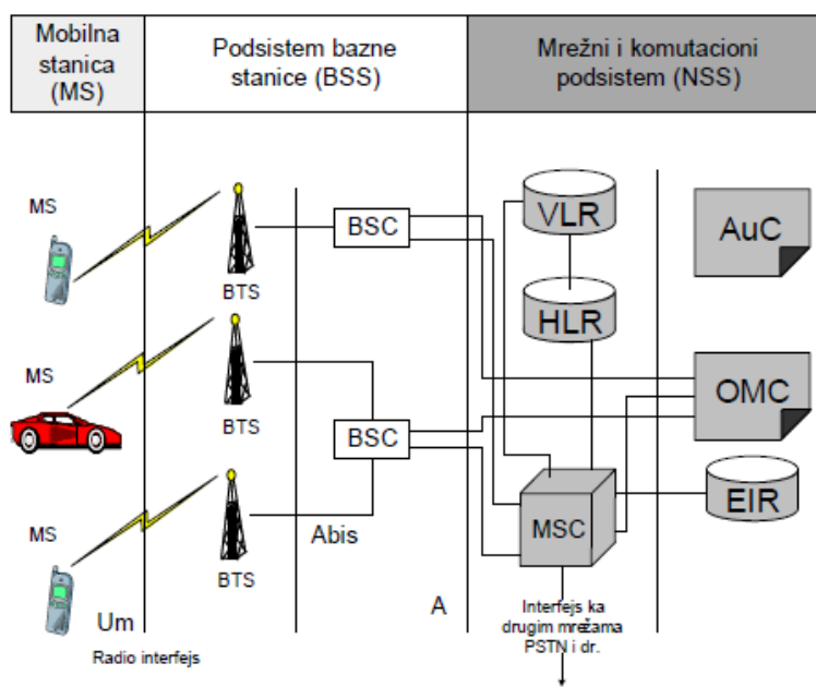
Slika 6.4. Arhitektura GSM sistema
